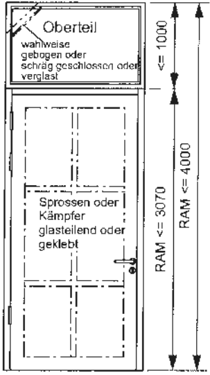
dargestellte Ansicht: Gangflügel DIN links: Gangflügel DIN rechts im Spiegelbild
